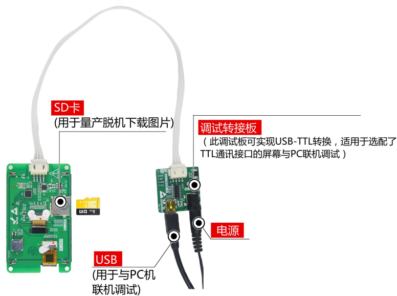
图 1-3 调试工具图
